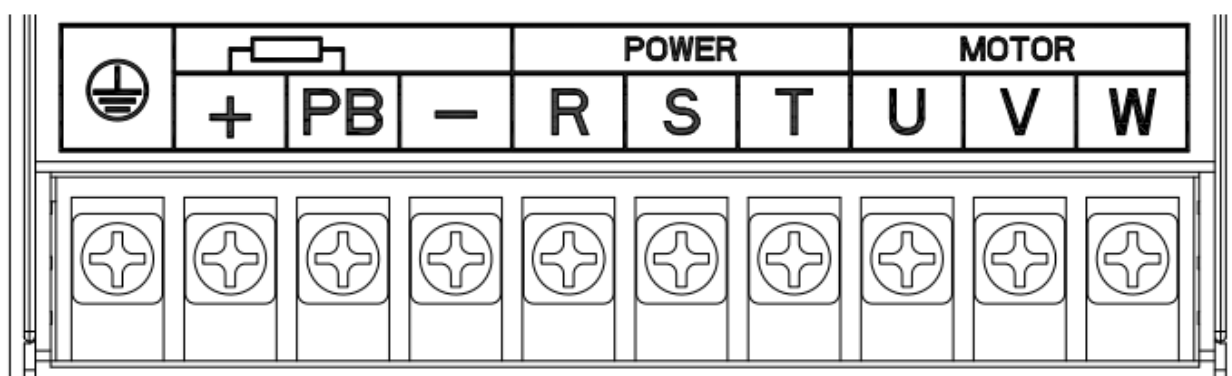
Рисунок 3 – Вид силовых клемм для VFD510-5R5GT4B
