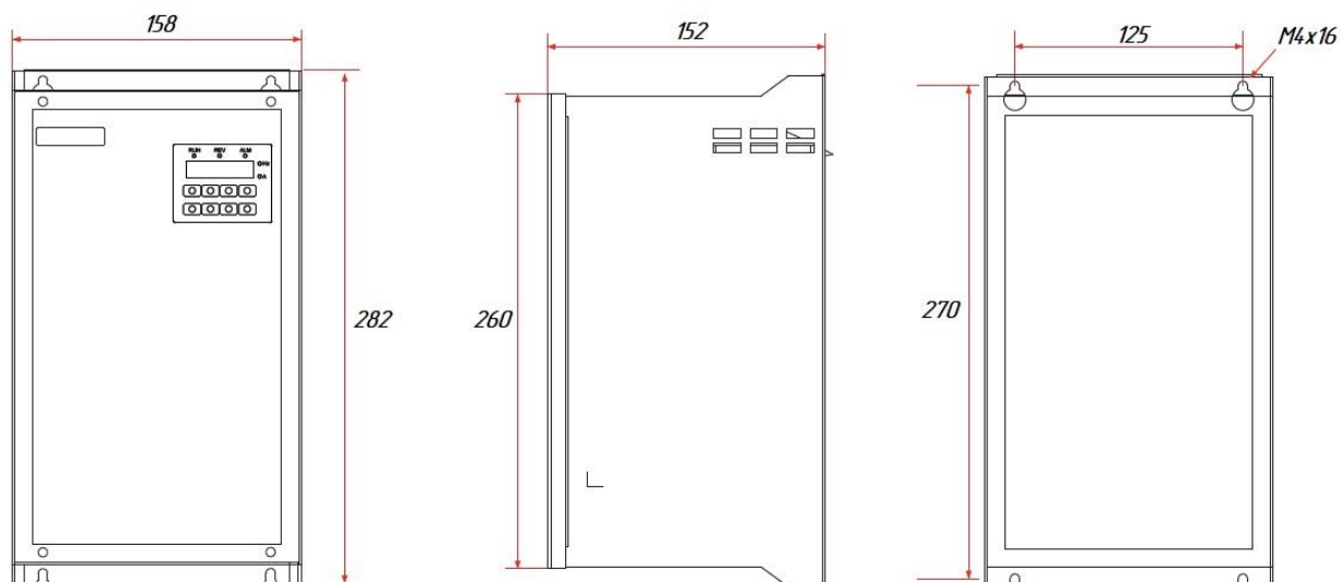
Рисунок 1 – габариты VFD510-5R5GT4B.
